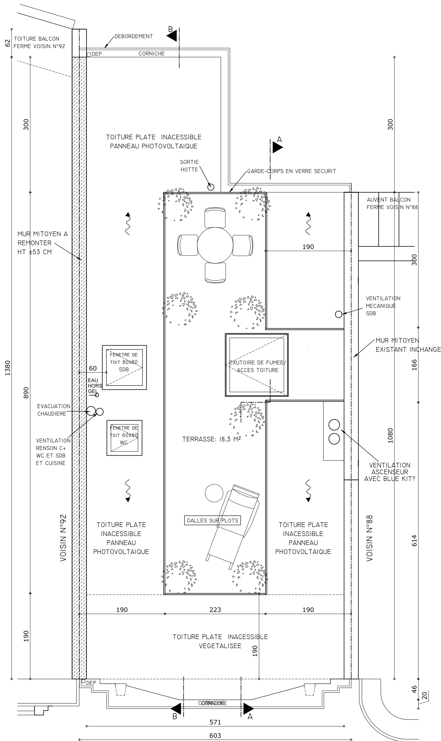
TOITURE : SITUATION PROJETEE
