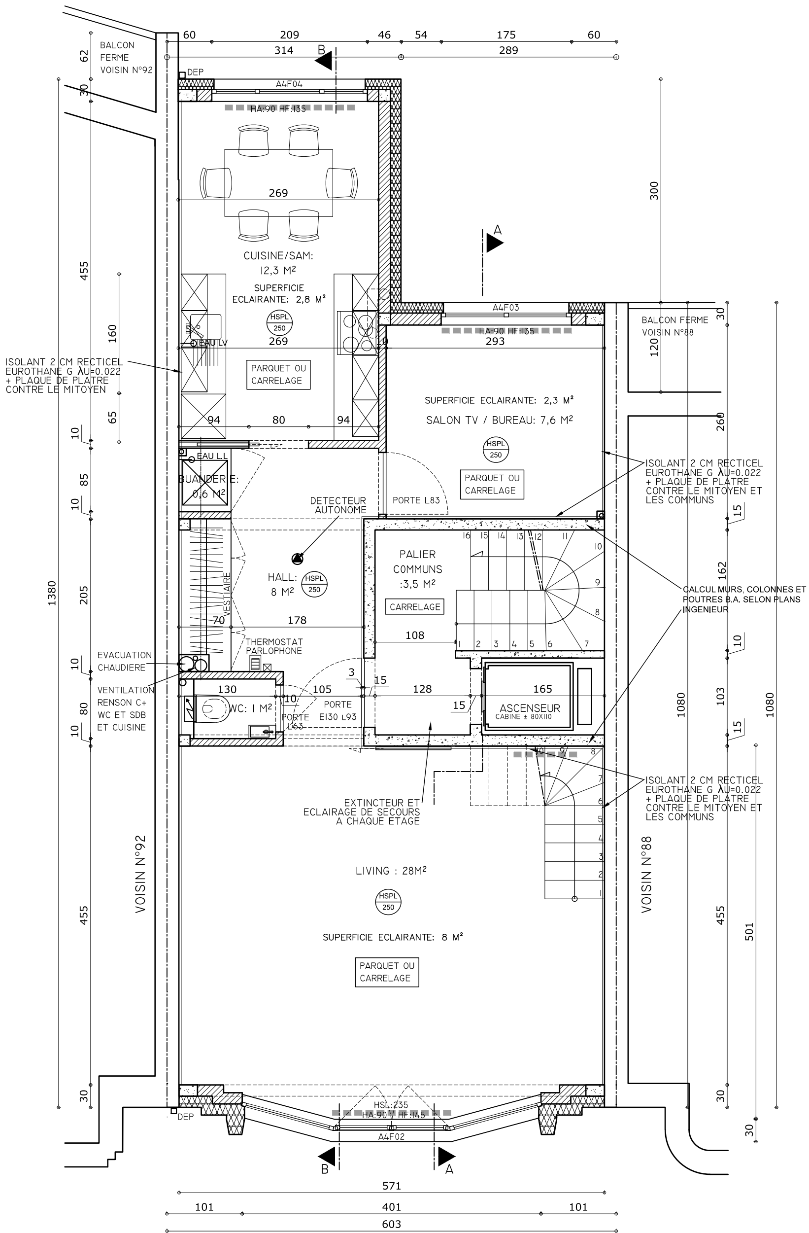
4EME ETAGE : SITUATION PROJETEE APPARTEMENT 4 - DUPLEX
