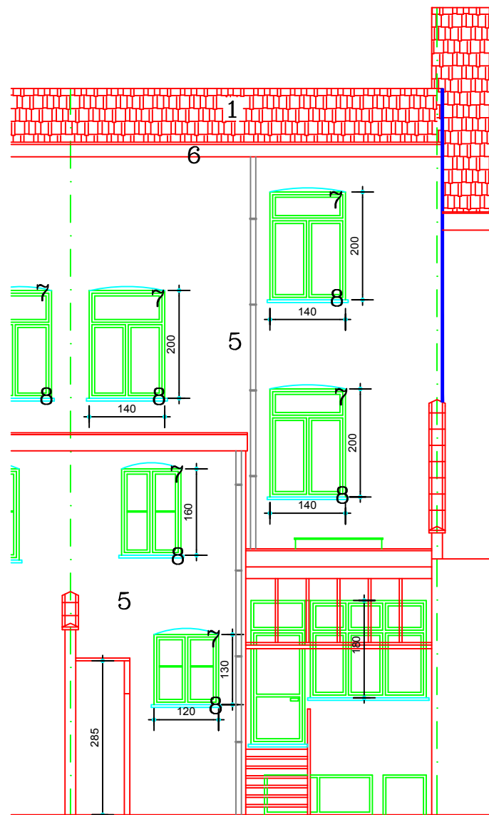
BT ACHTERGEVEL 1/100
