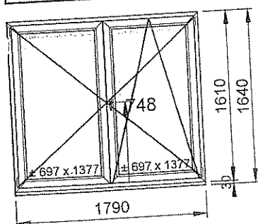
1/50 - Vue intérieure
