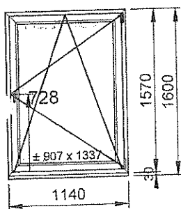
1/50 - Vue intérieure
