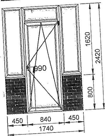
1/50 - Vue intérieure
