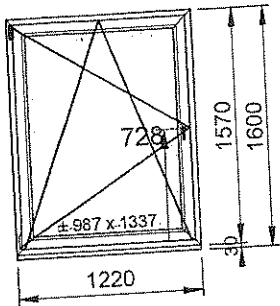
1/50 - Vue intérieure
