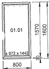
1/50 - Vue intérieure
