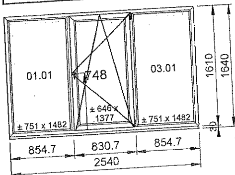
1/50 - Vue intérieure
