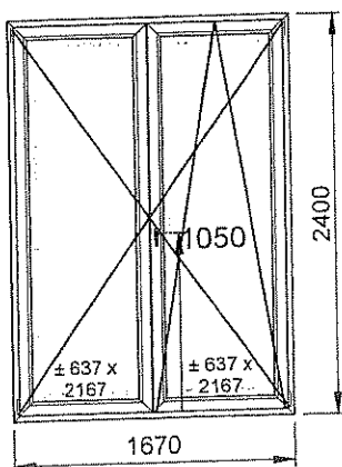
50 - Vue intérieure
