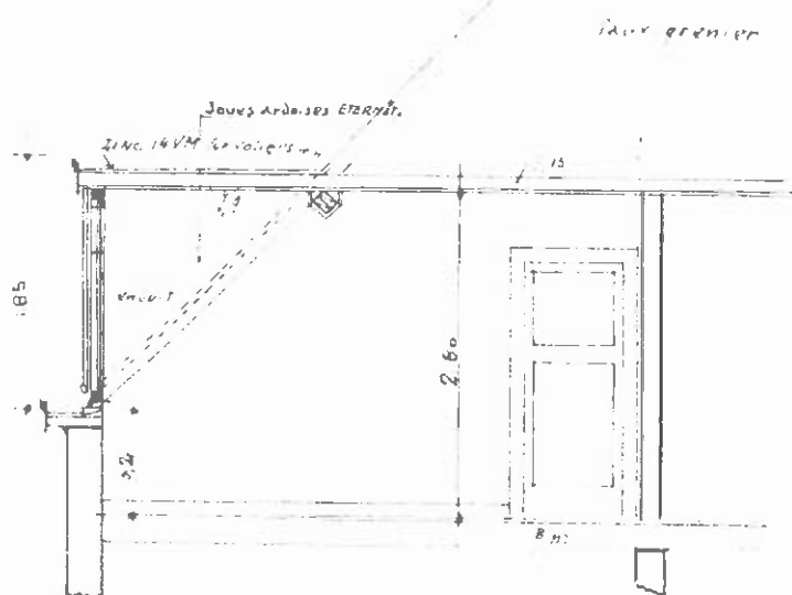
COUPE ETAT PROJETÉ
