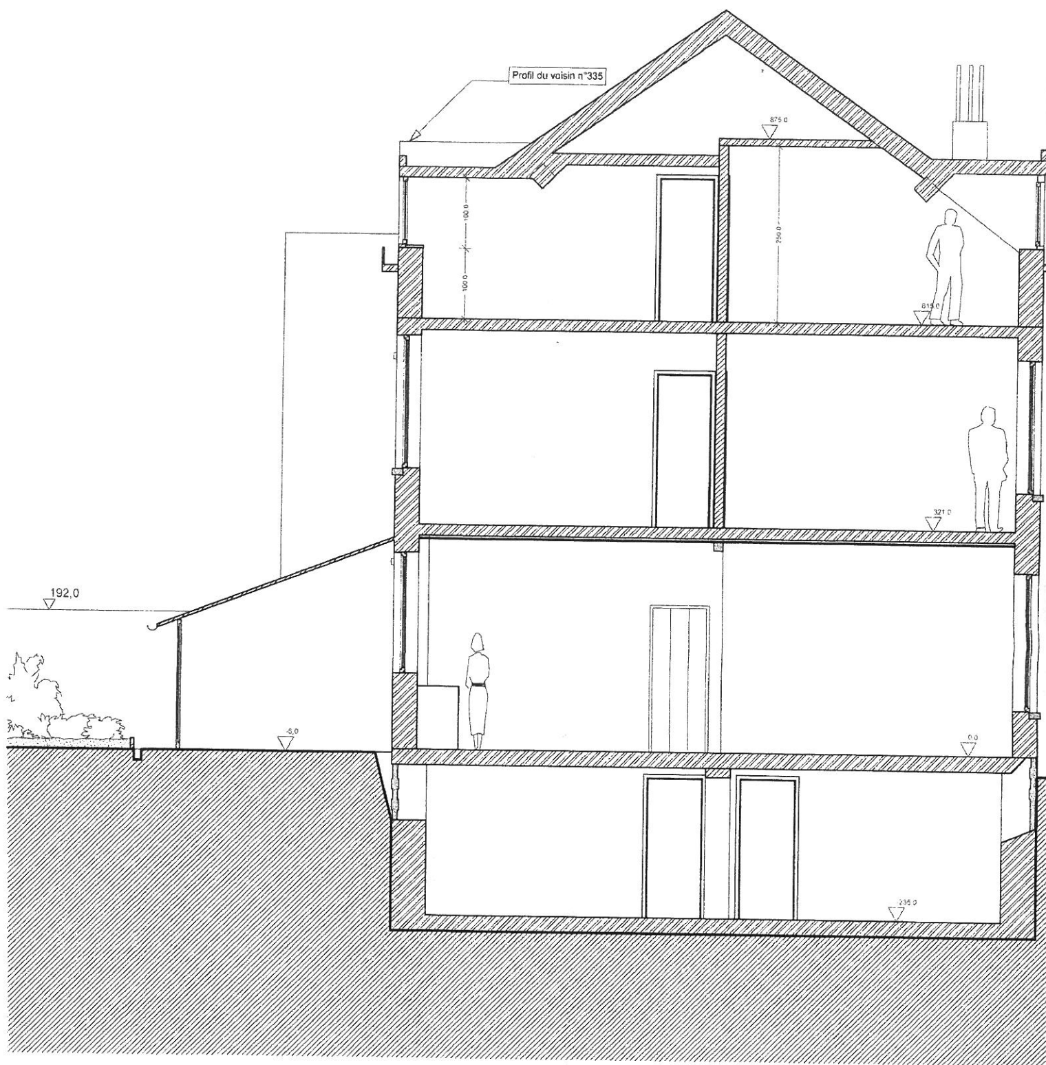
Coupe A-A'
