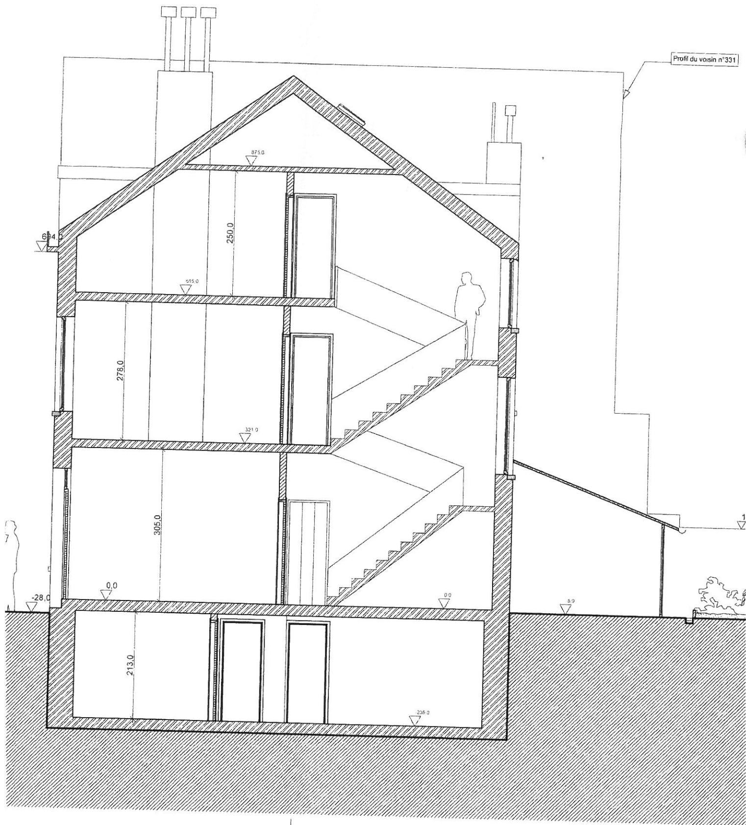
Coupe B-B'
